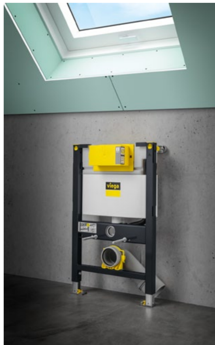
Niższe stelaże podtynkowe doskonale sprawdzą się np. w łazience na poddaszu
