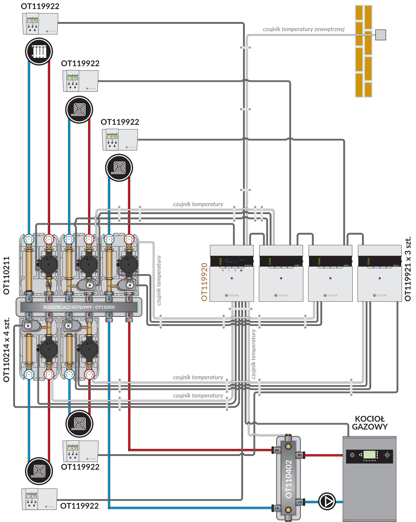
Schemat instalacji z zastosowaniem sprzęgła pionowego, systemu DN25 oraz sterowania obsługującego 5 pomp i 4 zawory z siłownikiem
