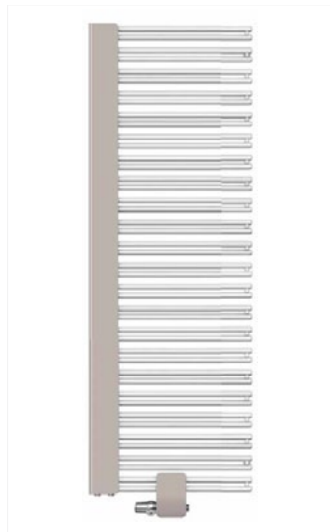
WIEDEŃ-VM SPA – jednostronnie otwarte kolektory grzewcze i proste, pionowe linie ramy dekoracyjnej połączone z nowoczesną technologią podłączenia środkowego czynią grzejnik designerskim elementem każdej łazienki. Model Wiedeń-VM SPA to przestronne miejsce do suszenia i wieszania tekstyliów czy ręczników. Wymiary: szer. 510, 610, 760 mm, wys. 1200, 1500, 1800 mm
