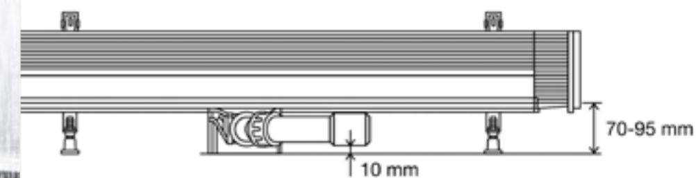
Wersja do remontowanych łazienek – wysokość 70 mm
